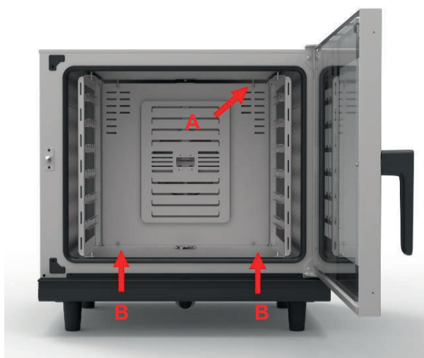
Rysunek 47. Śruby mocujące płytkę ssącą do COOK PRO
